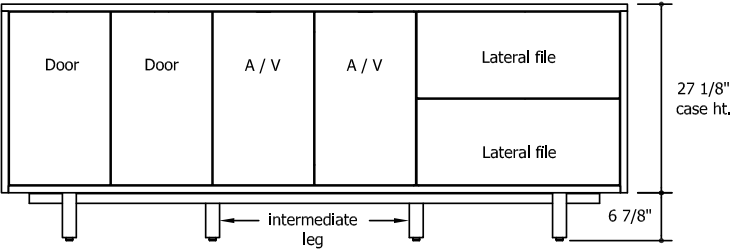
Buffet Height Credenza
